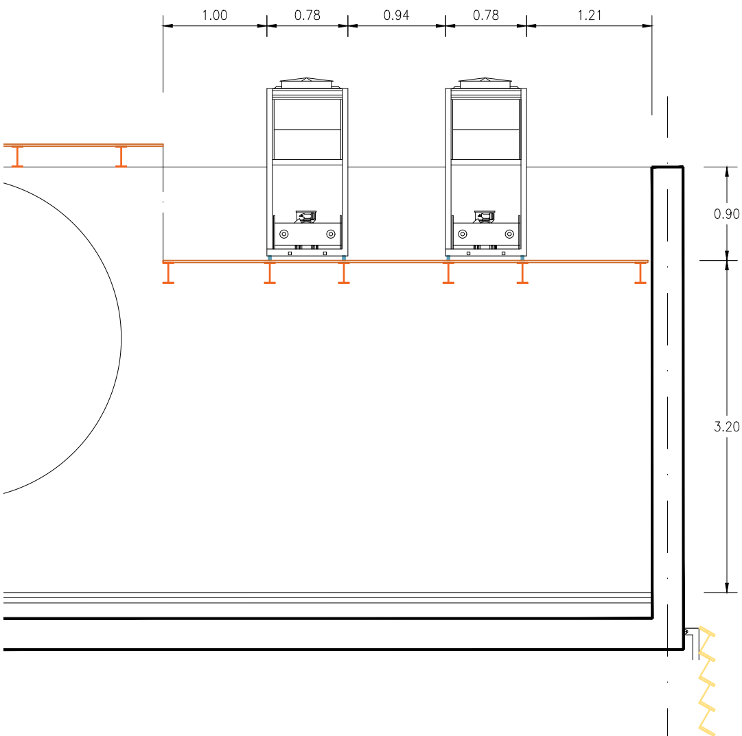
SECCIÓ - ESTRUCTURA ESCALA 1:50
