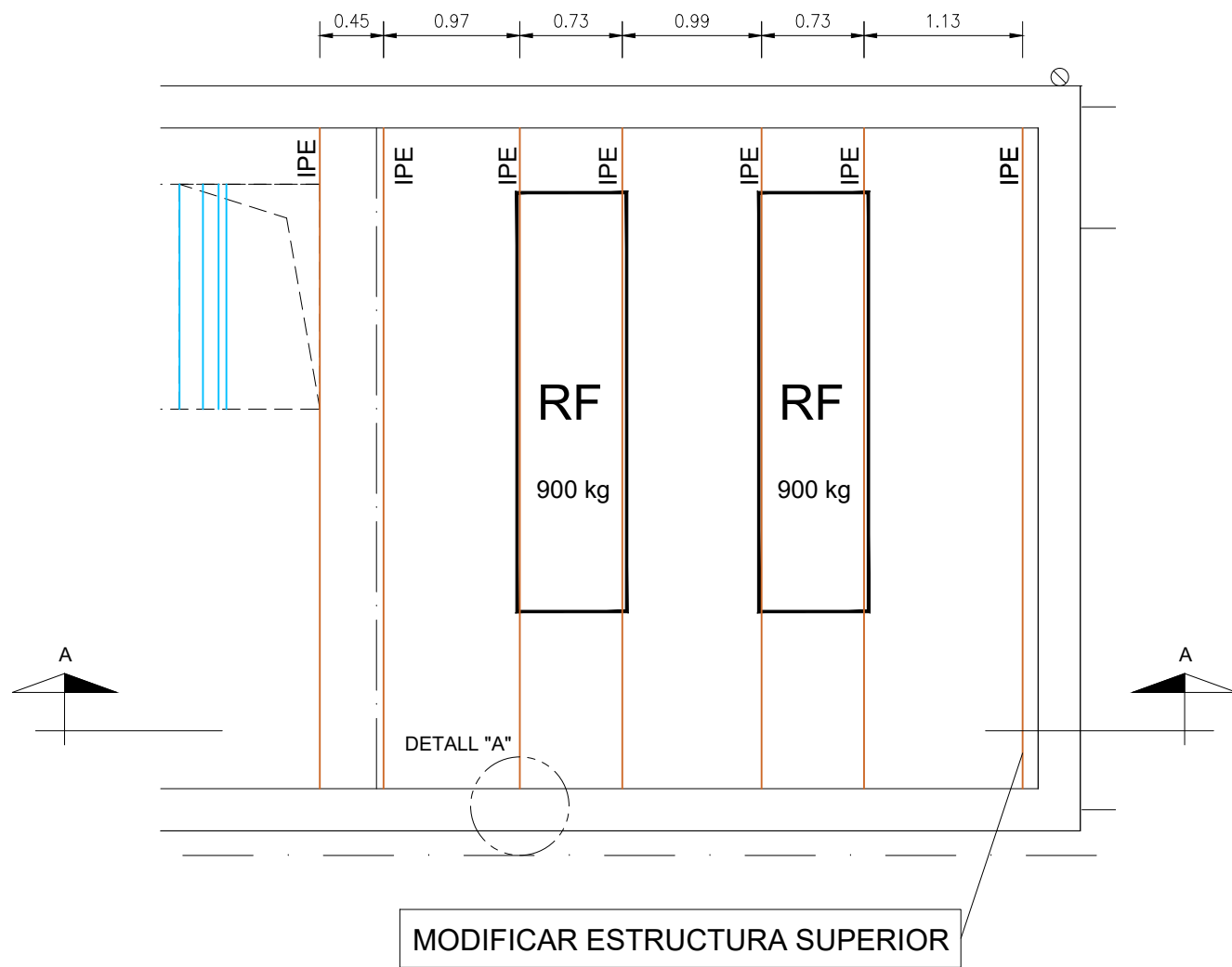
PLANTA - ESTRUCTURA ESCALA 1:50
