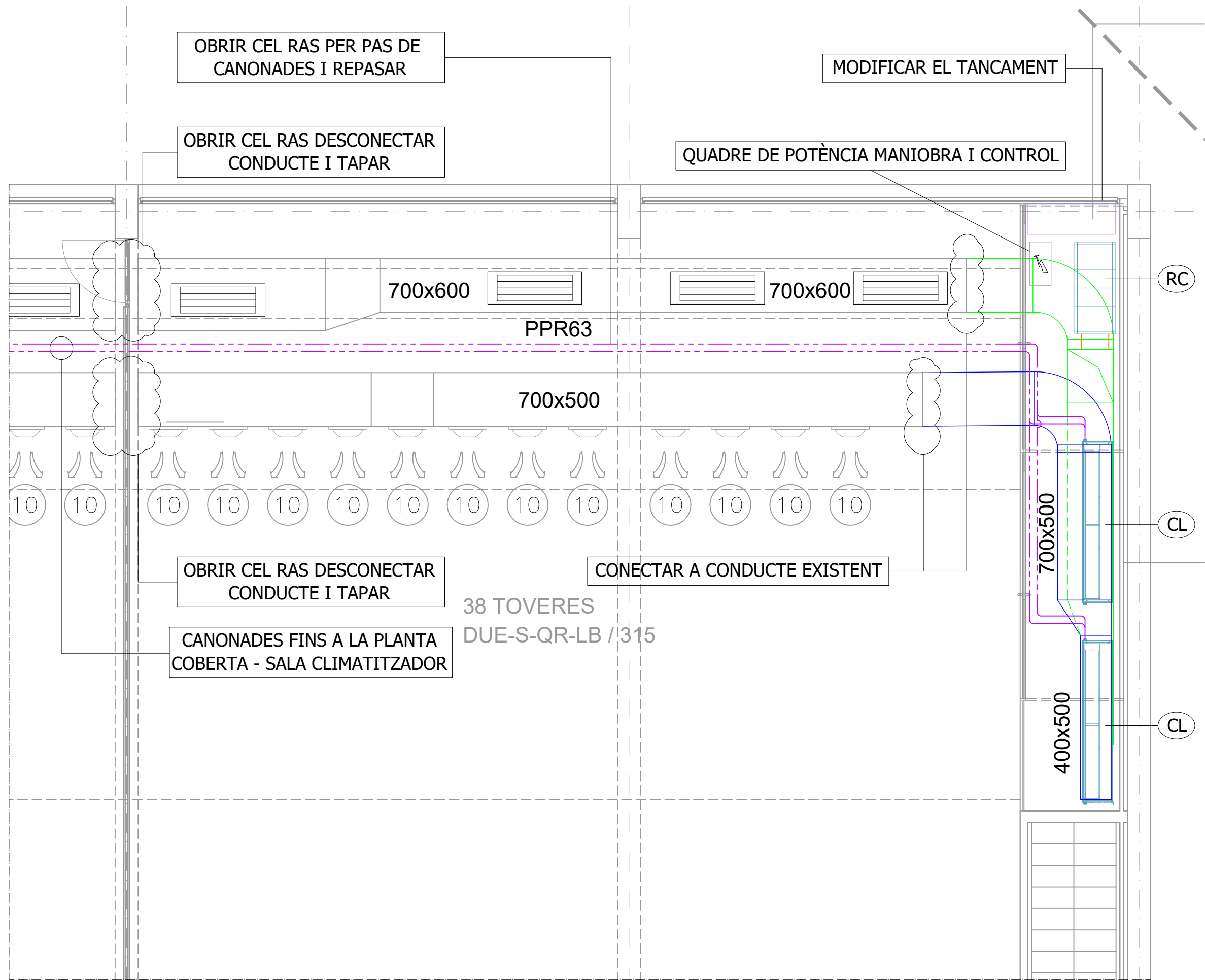
PLANTA GINNÀS - ESTAT REFORMAT
