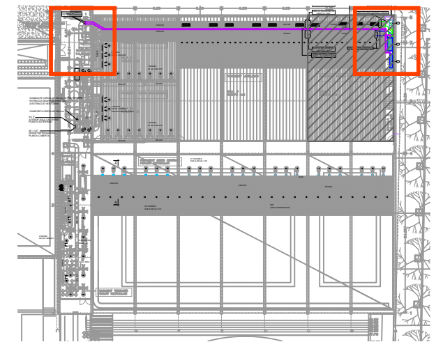
GINNÀS 3 - ESTAT REFORMAT (Canonades)
