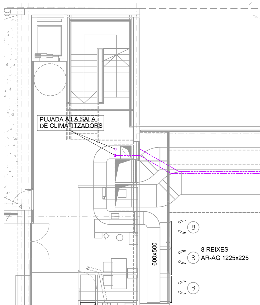
PLANTA 1 - ESTAT REFORMAT - CANONADES
