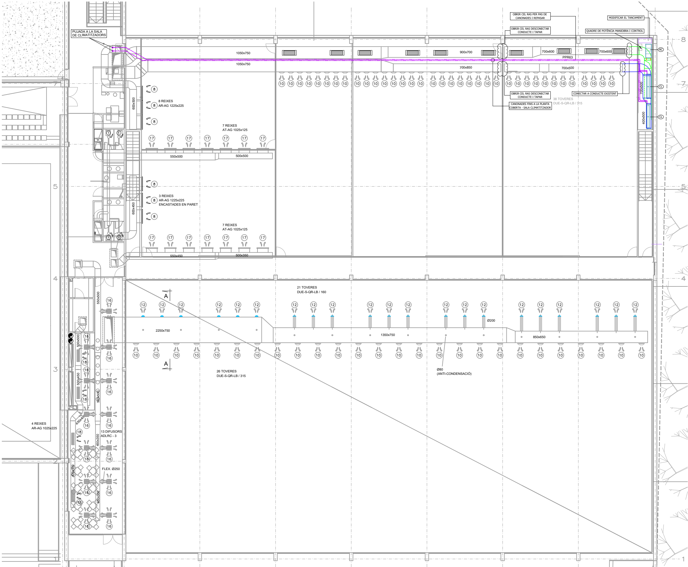
PLANTA GIMNÀS 3 - ESTAT REFORMAT - CANONADES CLIMATITZADORS
