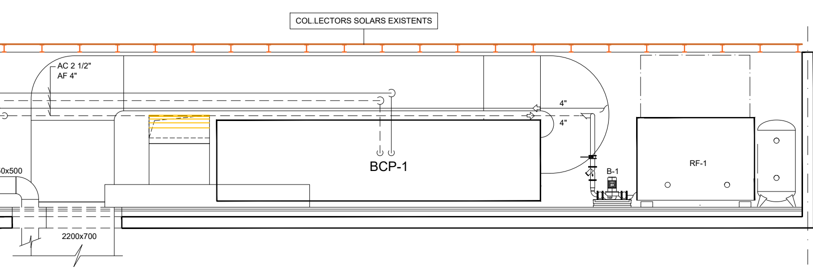
SECCIÓ A-A' - ESTAT ACTUAL
