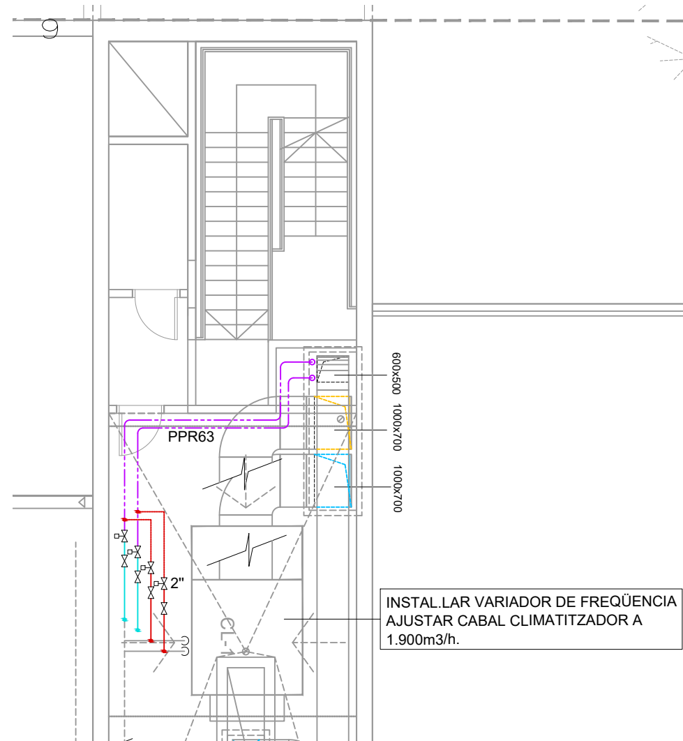
PLANTA COBERTA - ESTAT REFORMAT - CANONADES
