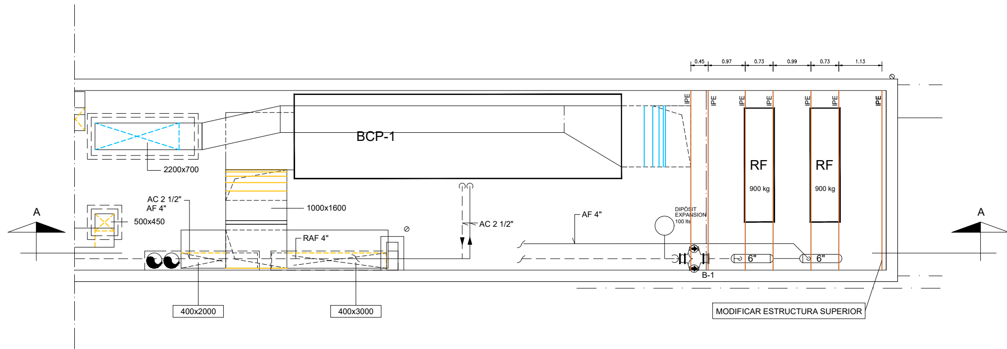
PLANTA - ESTAT REFORMAT
