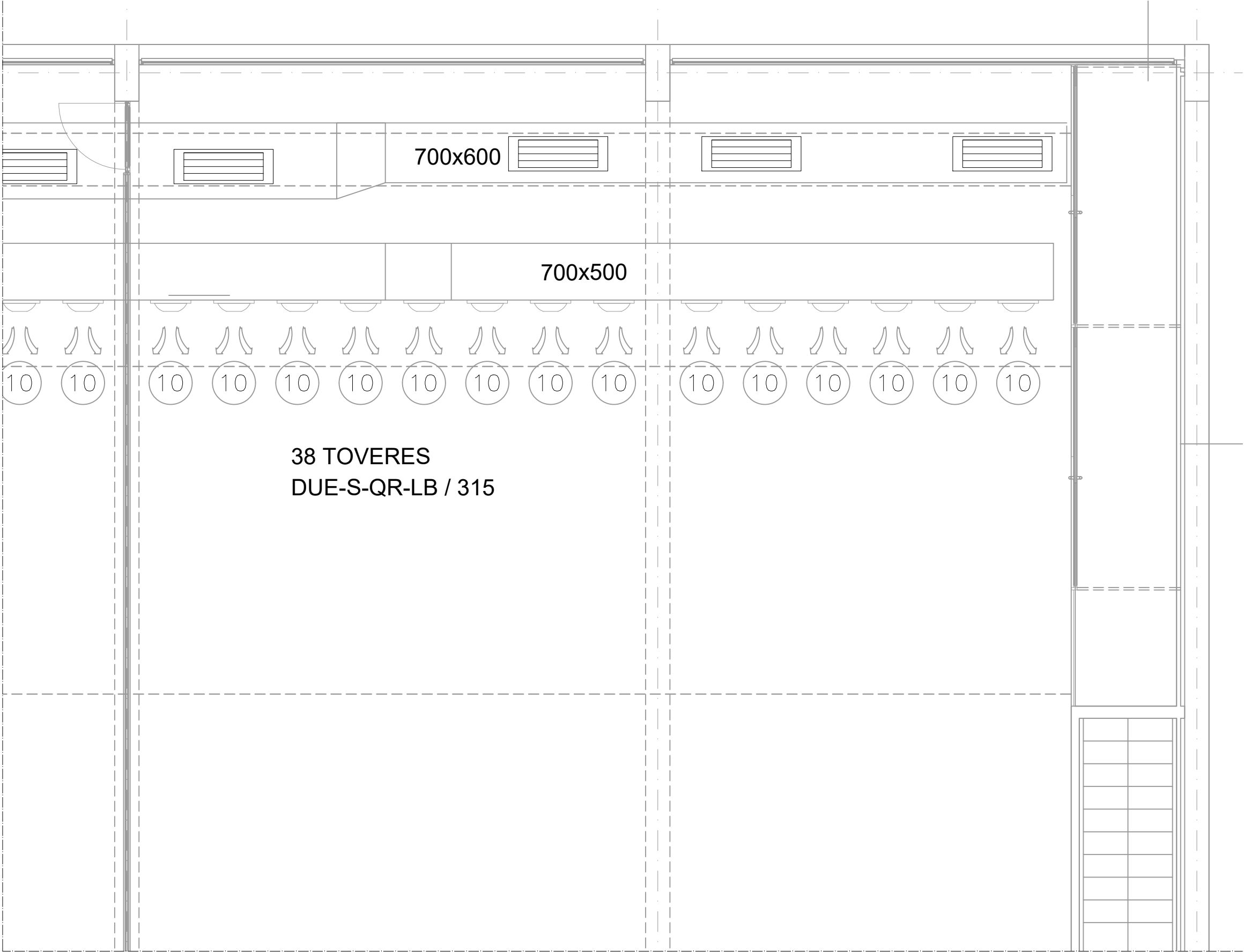
PLANTA GIMNÀS - ESTAT ACTUAL
