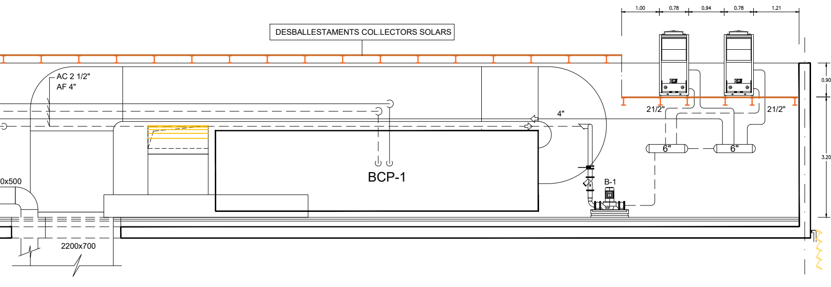
SECCIÓ A-A' - ESTAT REFORMAT
