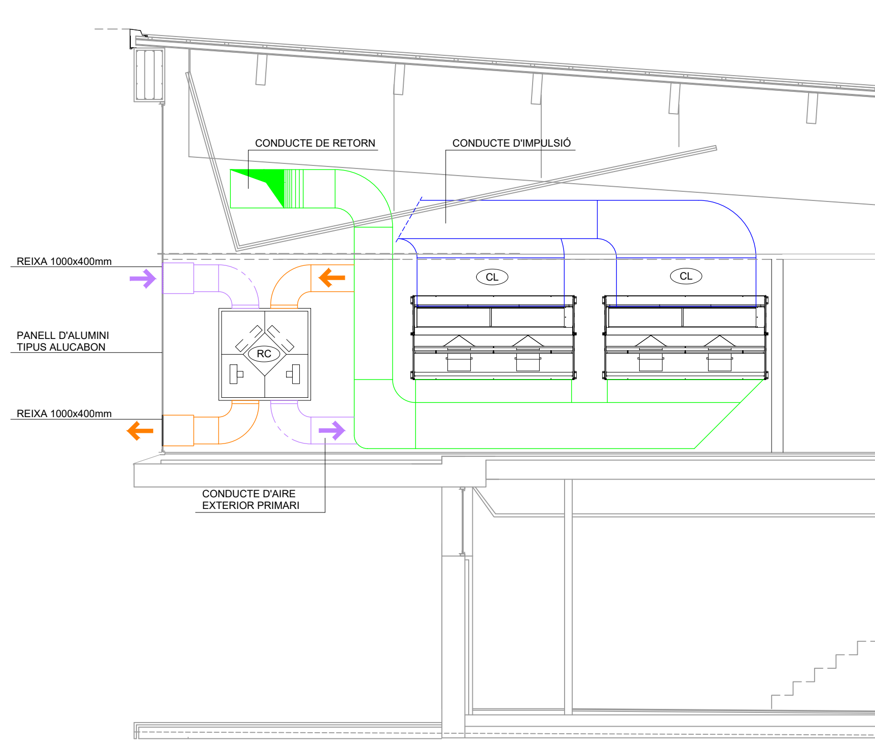
SECCIÓ GIMNÀS 3 - ESTAT REFORMAT
